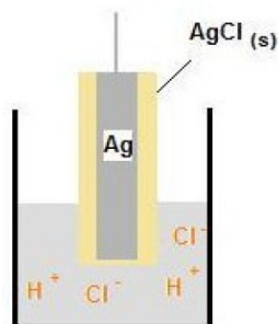
Rys. 4. Schemat półogniwa chlorosrebrowego.
